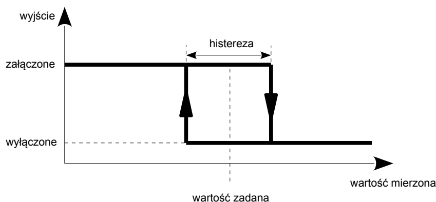
Rysunek 10. Sposób działania wyjścia typu grzanie
