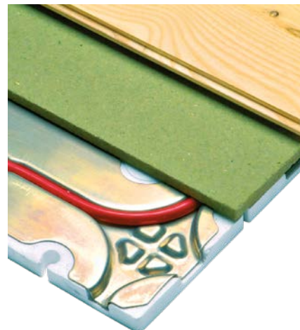
Widok warstw podłogi z ułożoną płytą DEVIcell Dry™
