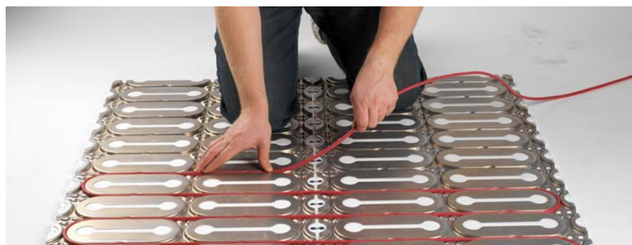
Sposób montażu kabla grzejnego z użyciem płyty DEVIcell Dry™
