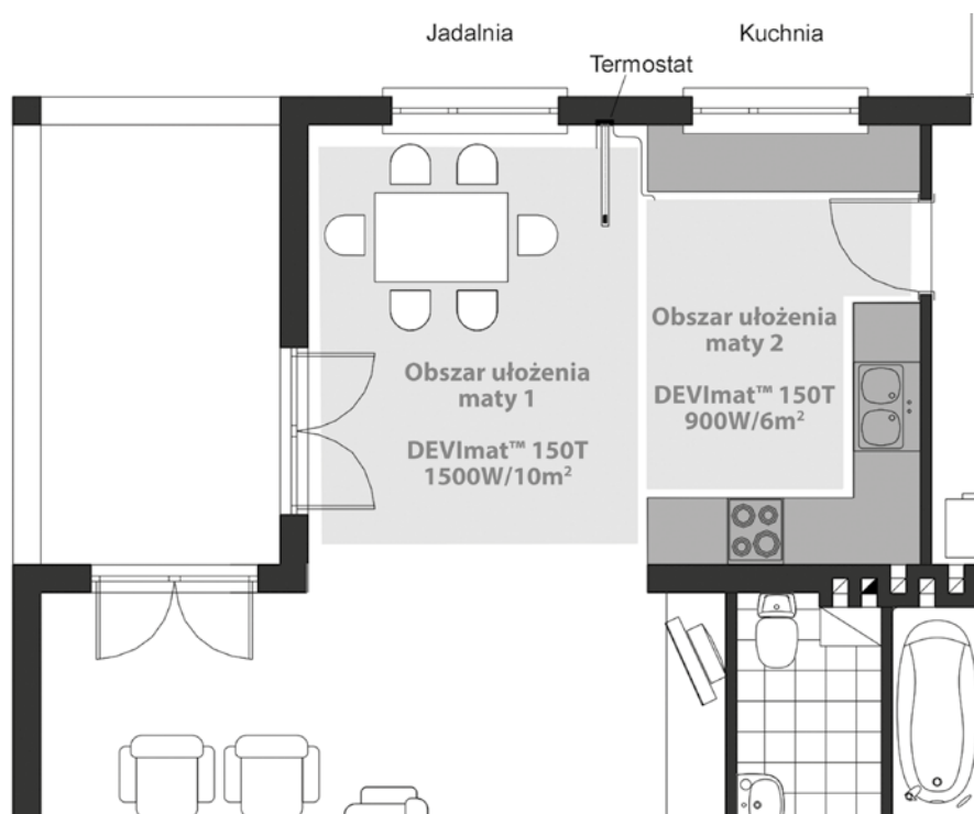
Przykładowy sposób rozmieszczenia i sterowania matami DEVImat™ 150T
