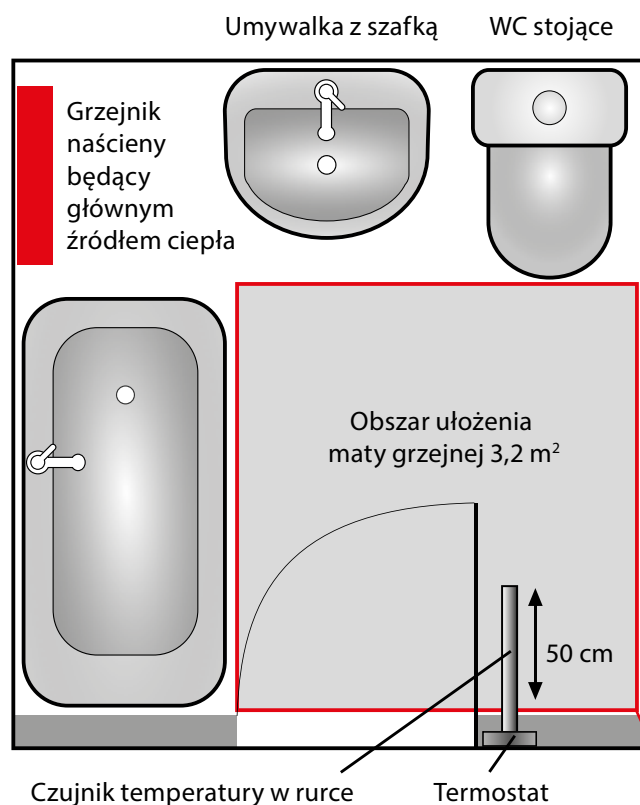
Mata grzejąca DEVI ® mat™ 150T do podłóg kamiennych
