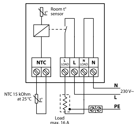
Schemat DEVireg™ Touch
