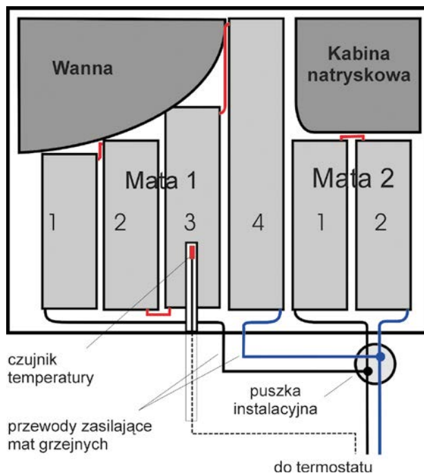
Przykładowe połączenie dwóch mat DEVIheat™ 150S
