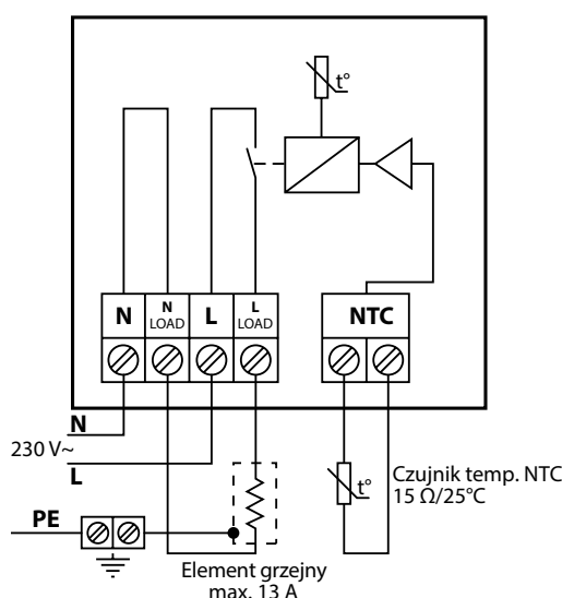
Schemat DEVireg™ Opti
