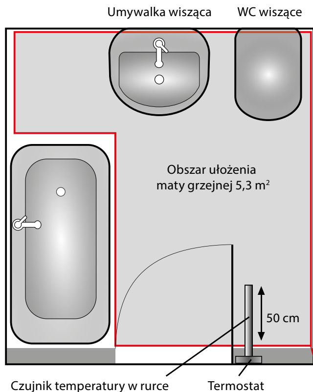
Mata grzejna DEVImat™ 150T do podłóg kamiennych
