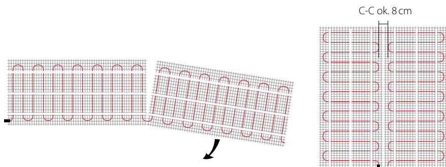
Układanie maty grzejnej wokół obszaru nieogrzewanego.
