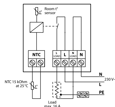
Schemat DEVlreg™ Smart
