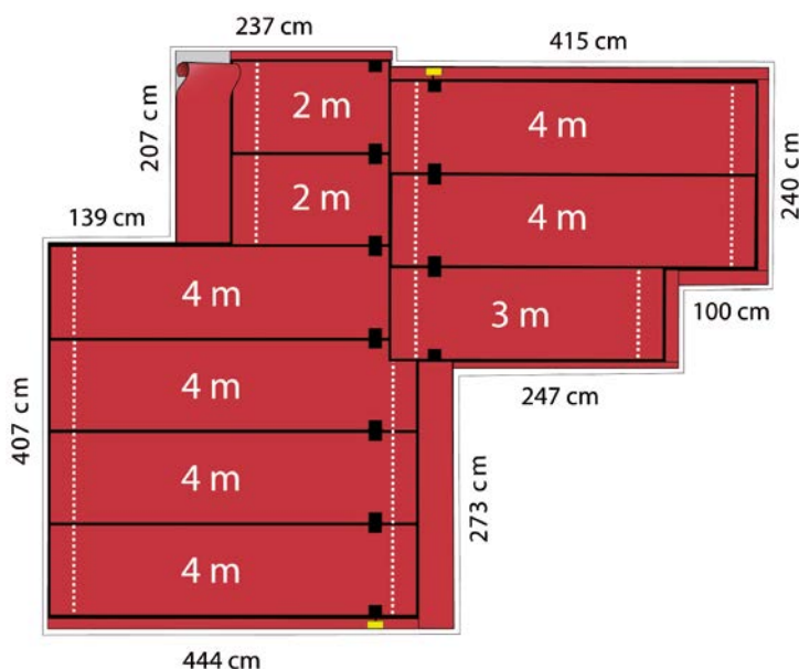
Przykładowe rozmieszczenie mat DEVIdry™
