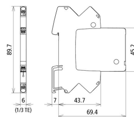
Rysunek wymiarowy BCO ML2 BE 24
