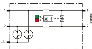
Schemat połączeń BCO CL2 BD 24
